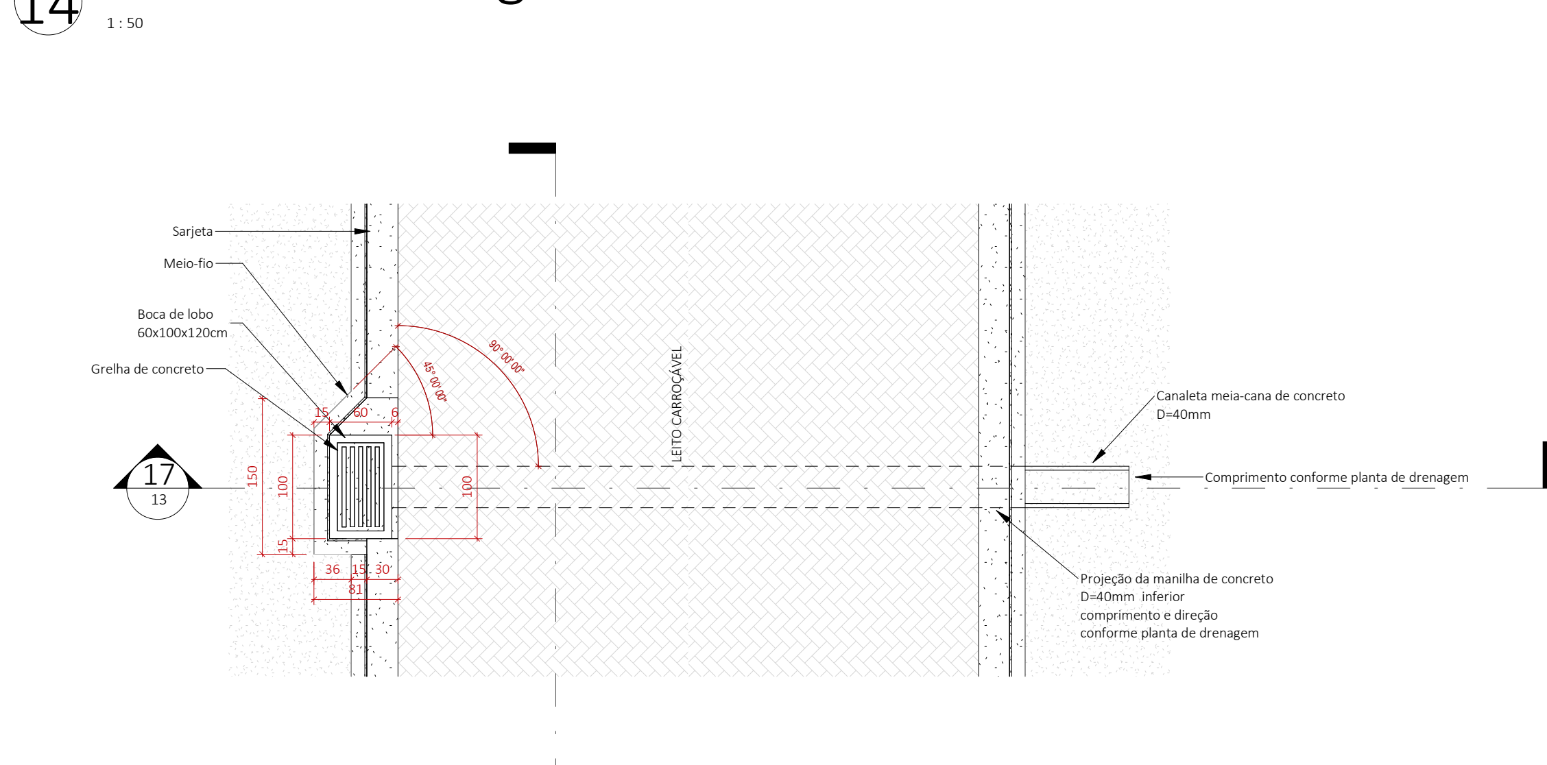
15 DET 14 - Drenagem
