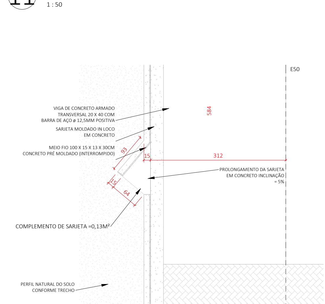
12 DET 11- Drenagem
