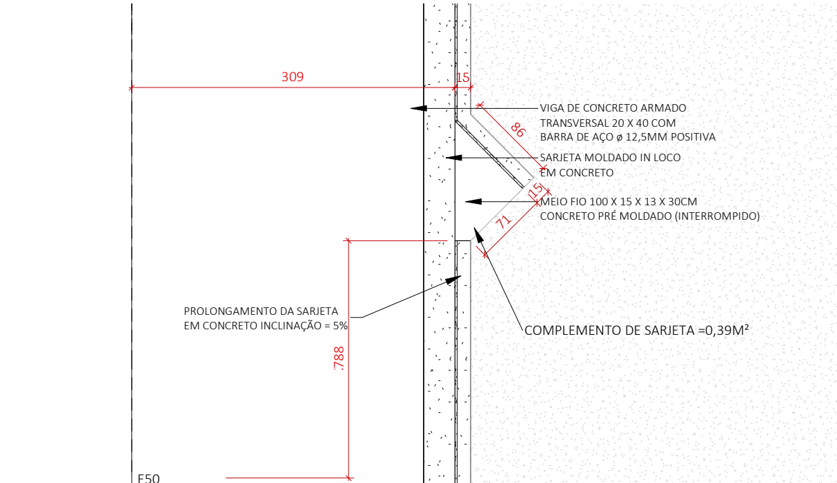
11 DET 10 - Drenagem
