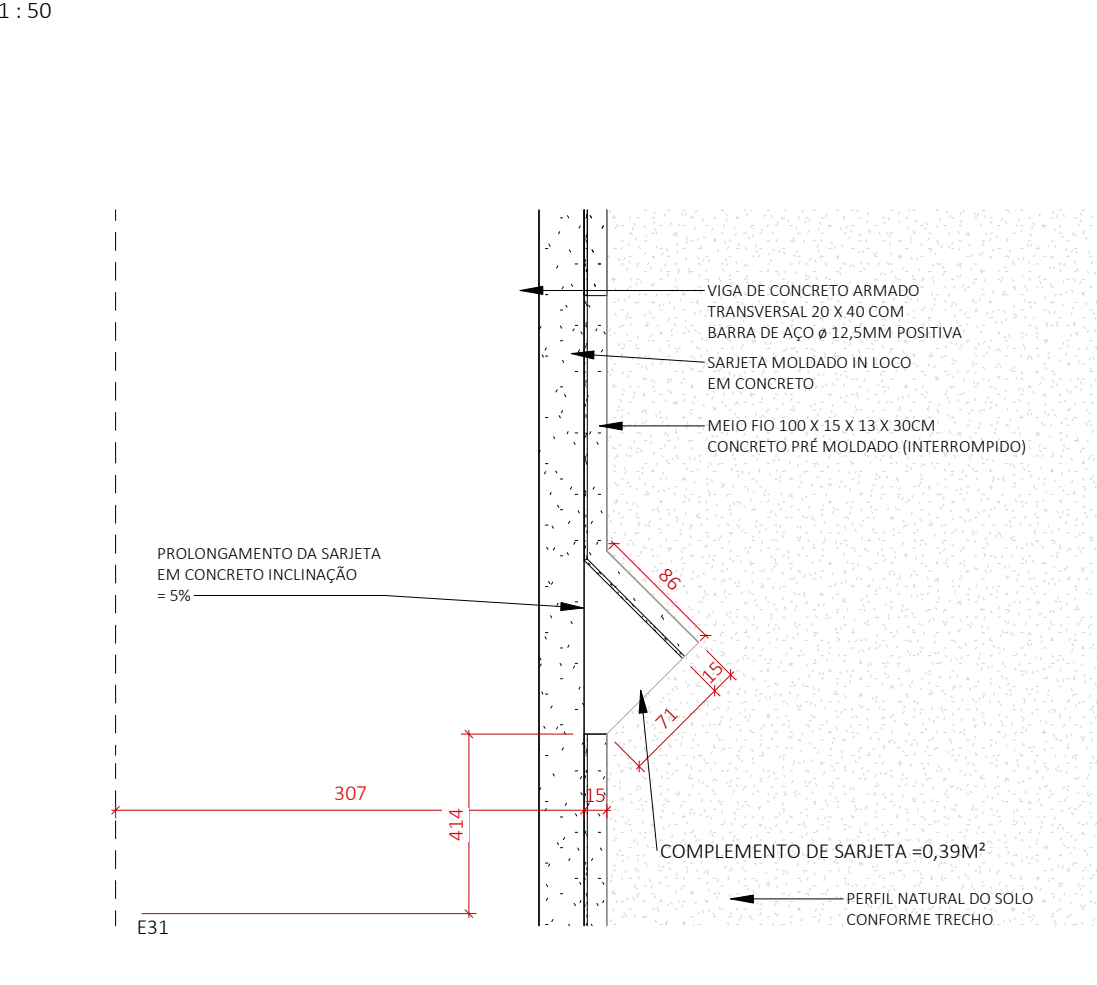
7 DET 06- Drenagem
