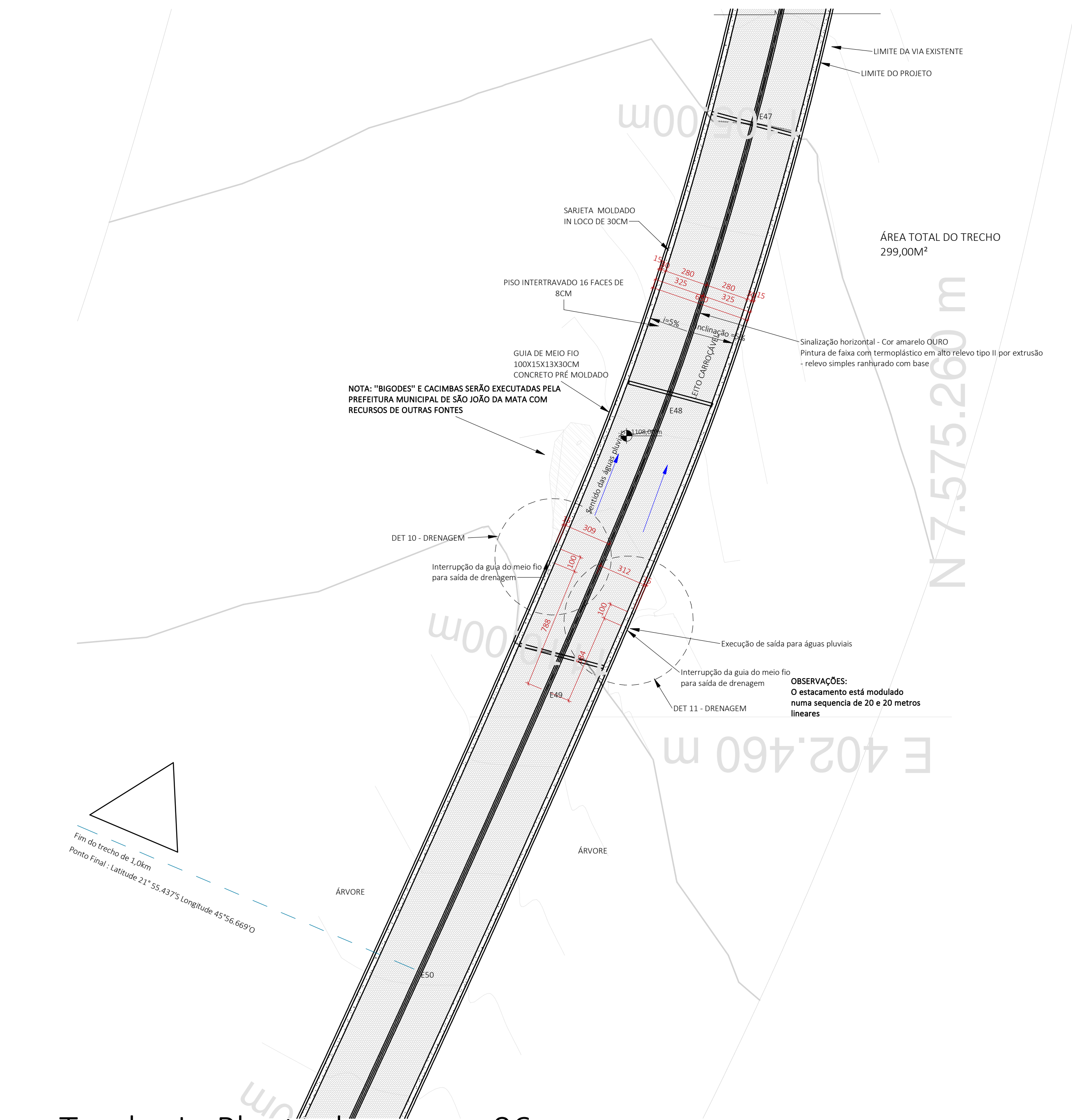
1 Trecho I - Planta drenagem 06
