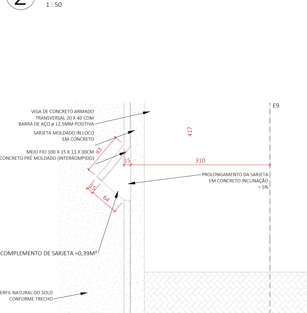
3 DET 02- Drenagem
