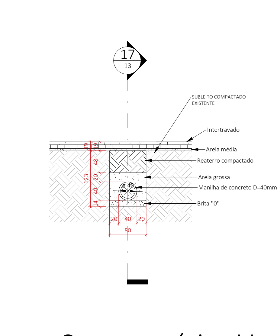
16 Corte genérico V
