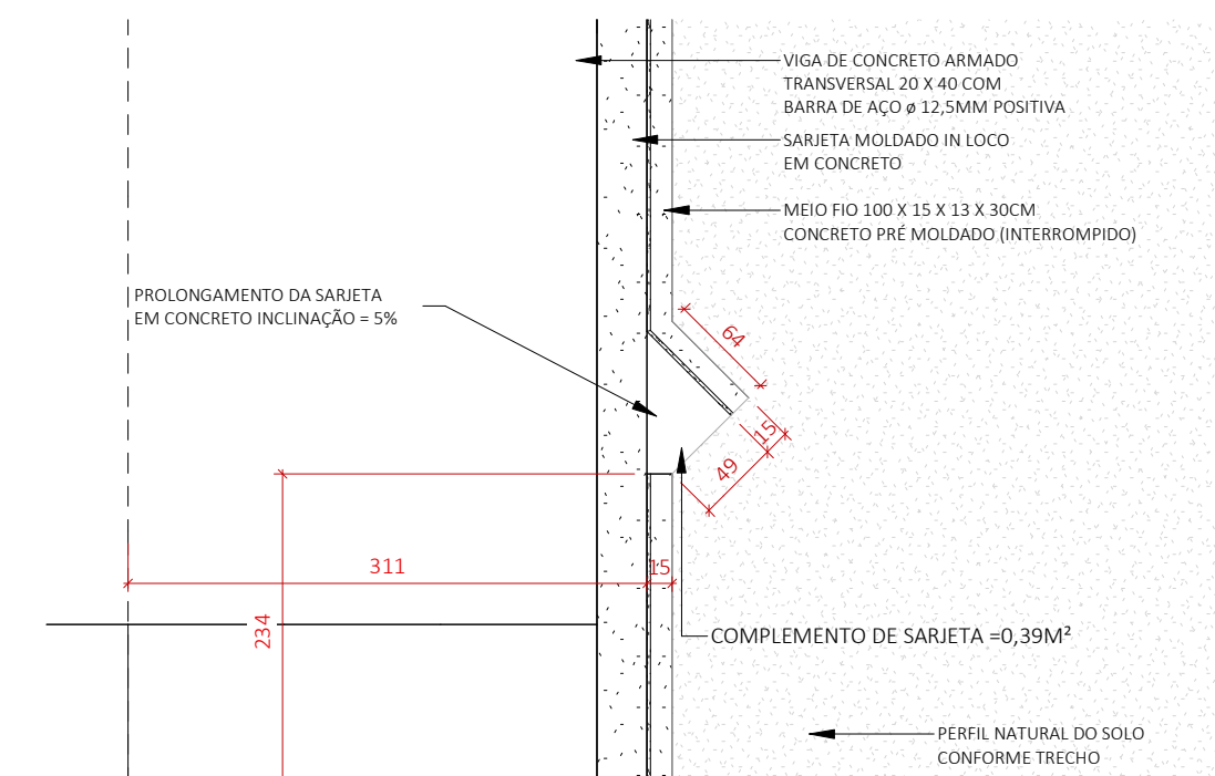
5 DET 04 - Drenagem
