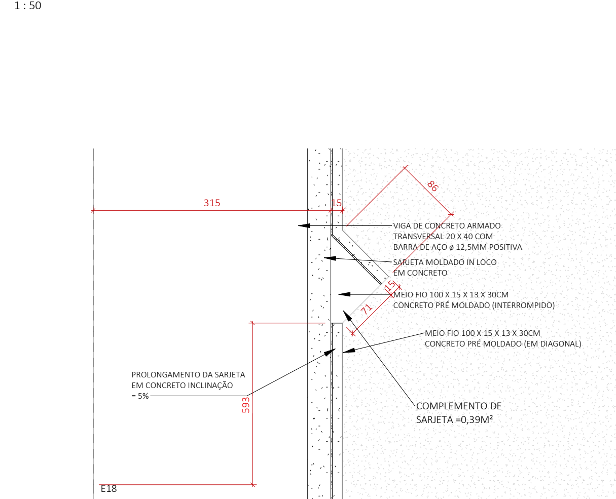
4 DET 03- Drenagem
