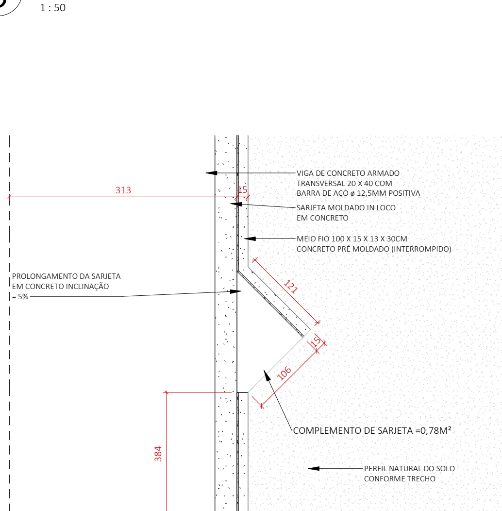
6 DET 05- Drenagem
