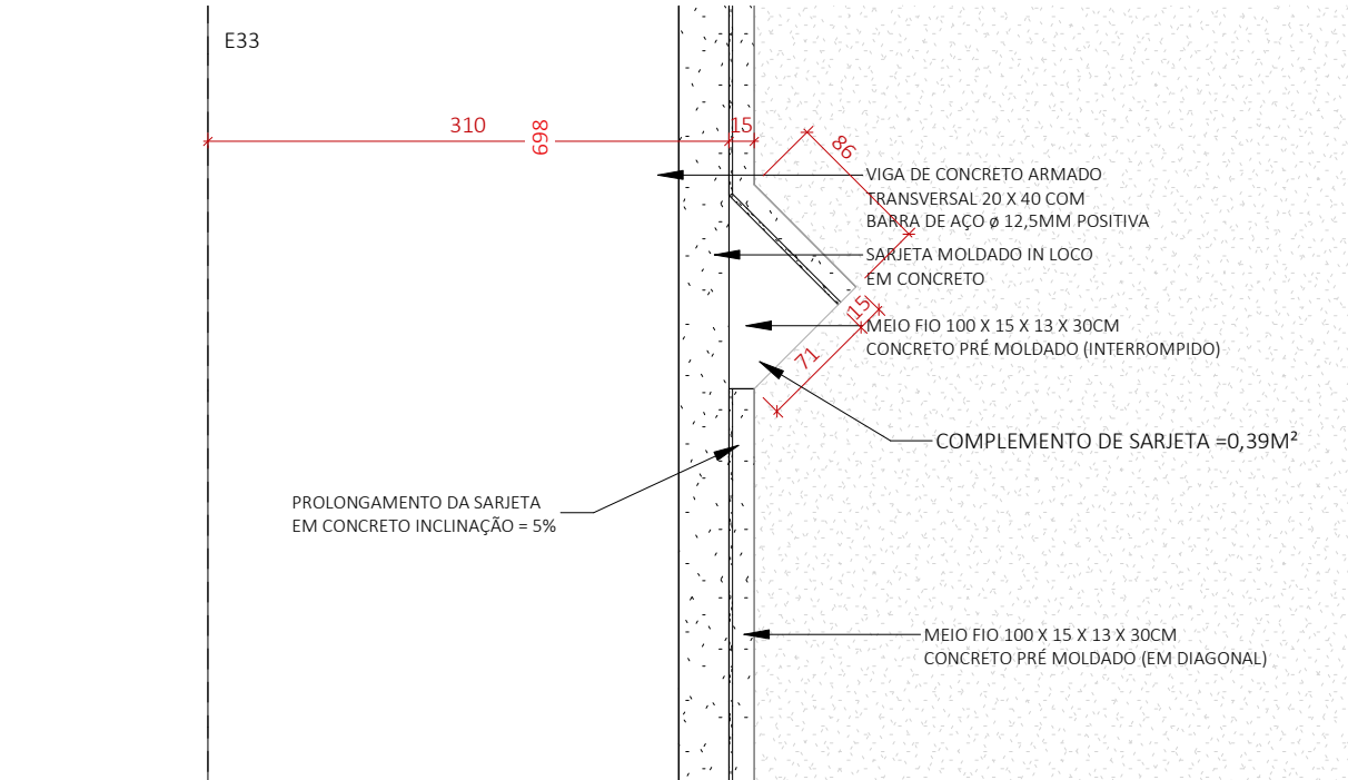
8 DET 07 - Drenagem
