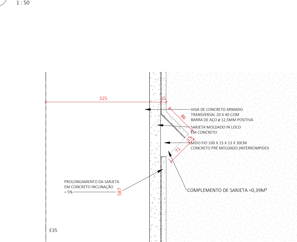
10 DET 09 - Drenagem
