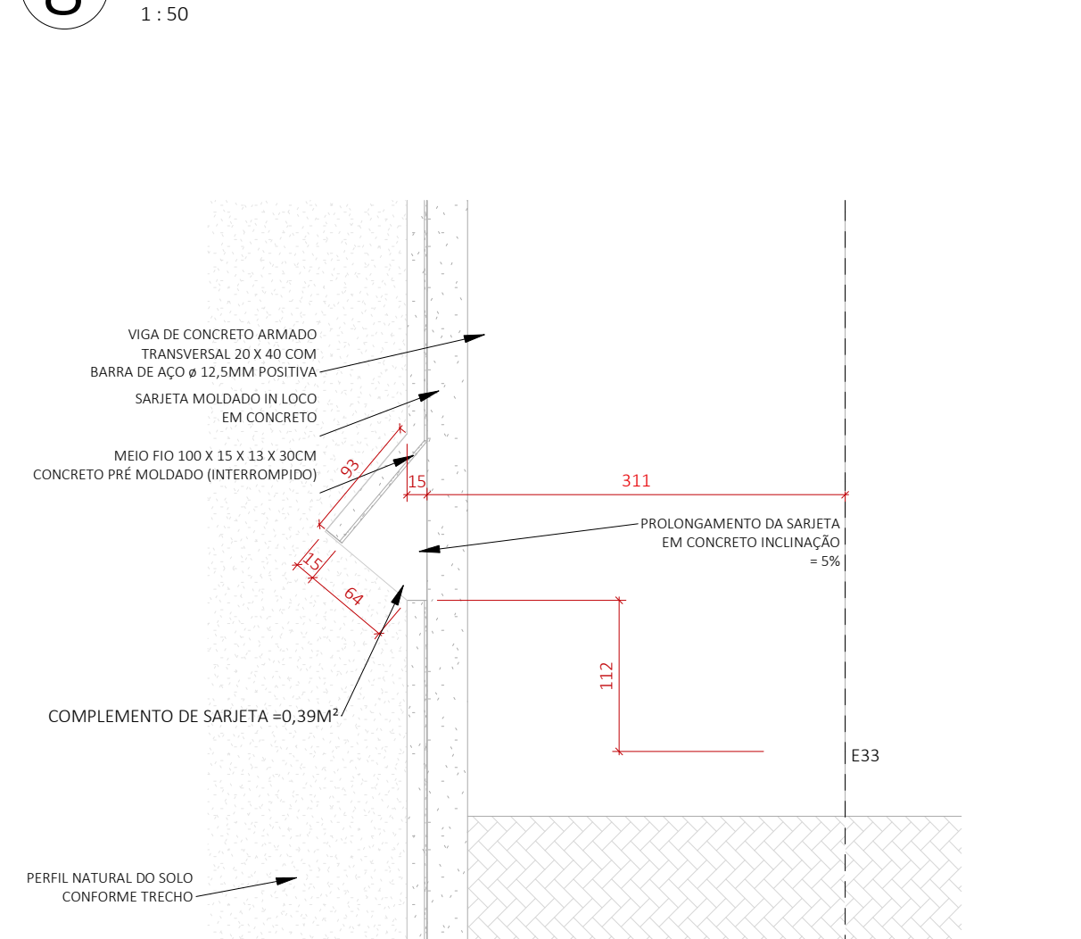
9 DET 08- Drenagem
