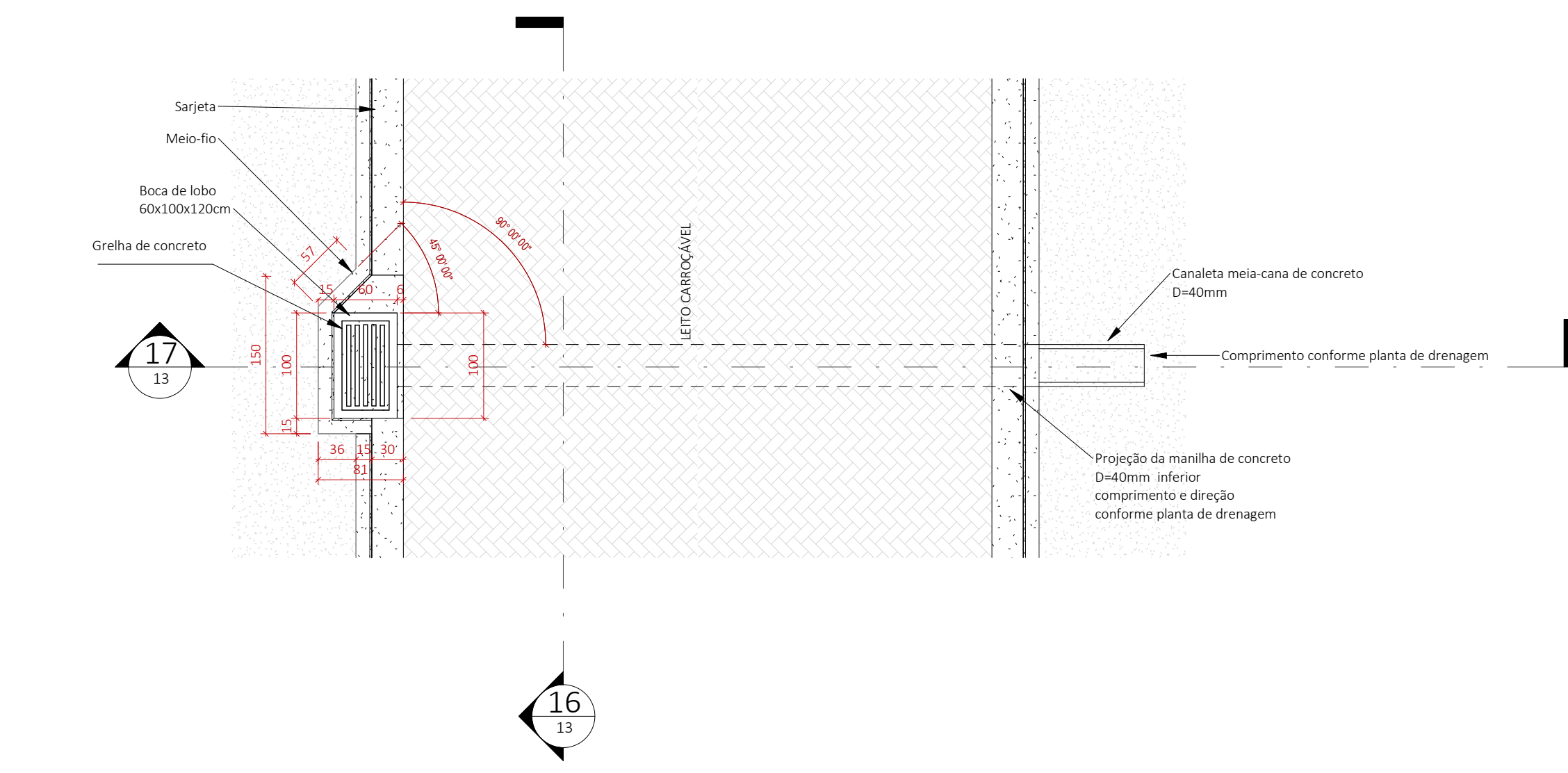
14 DET 13 - Drenagem
