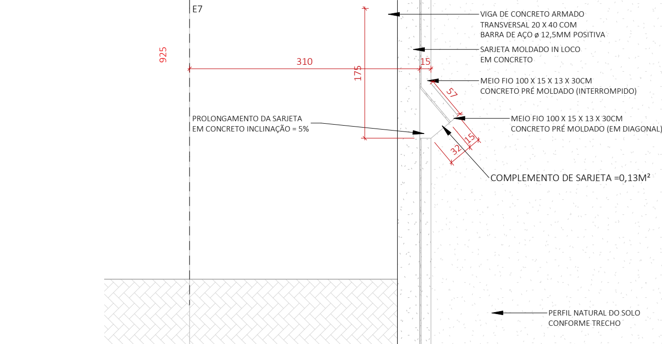
2 DET 01 - Drenagem
