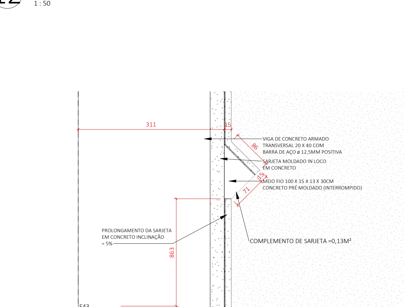
13 DET 12 - Drenagem
