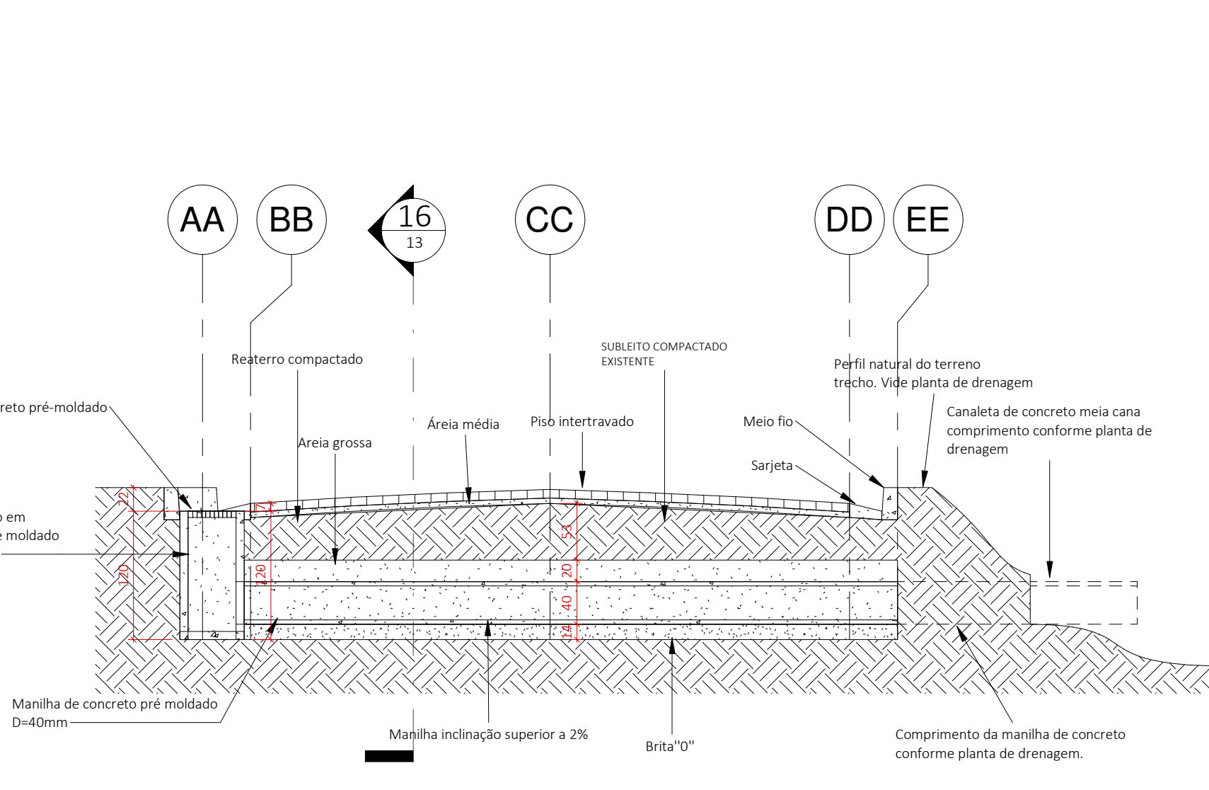
17 Corte genérico VI
